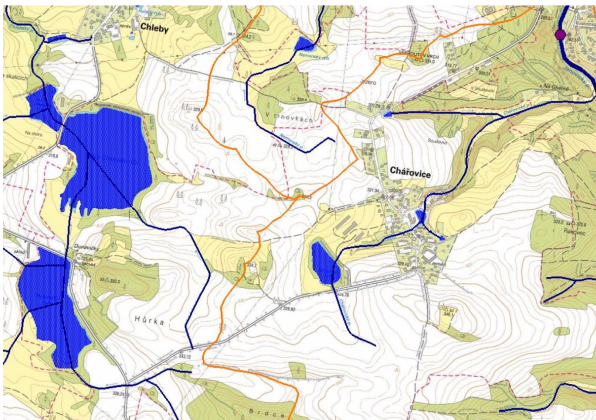
MAPA 4 HRANICE HYDROLOGICKÉHO POVODÍ 3. ŘÁDU (ORANŽOVÉ LINIE), VODNÍ TOKY A VODNÍ NÁDRŽE
